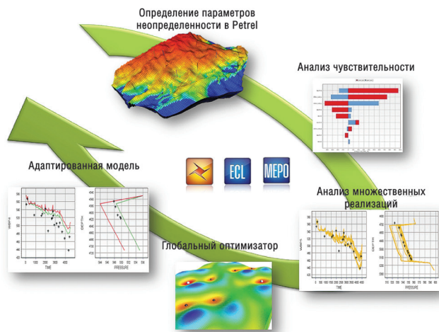
Рис. 3. Рабочий процесс по автоадаптации замеров пластового давления (XPT)
