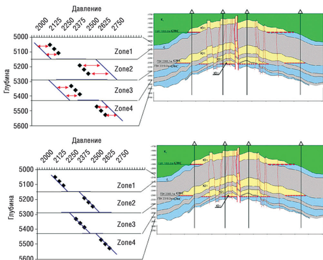
Рис. 2. Концепция адаптации замеров пластового давления (MDT/RFT/XPT): до адаптации (сверху), после адаптации (снизу)
